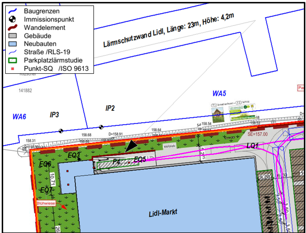
Abbildung: modifizierte Lärmschutzwand an Anliefergebäude
